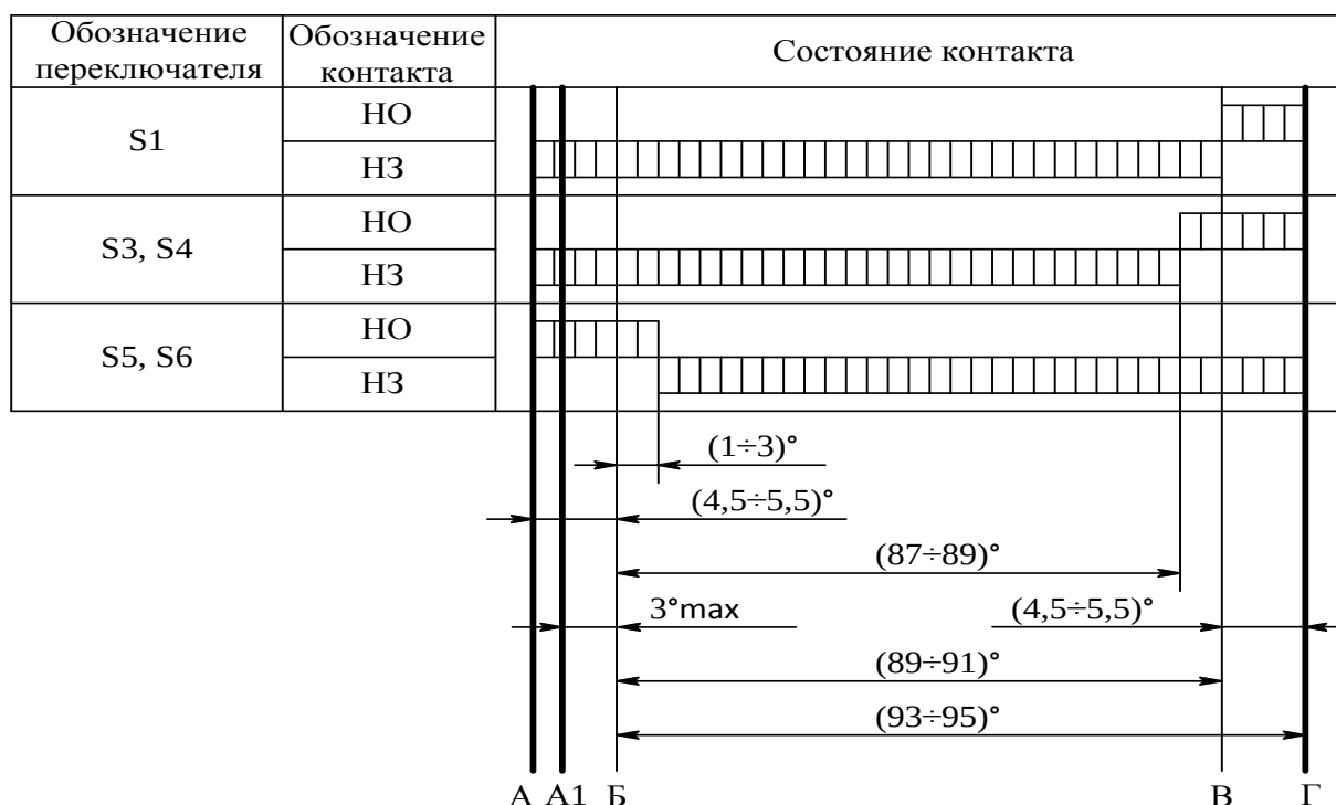
Циклограмма работы микропереключателей механизма
