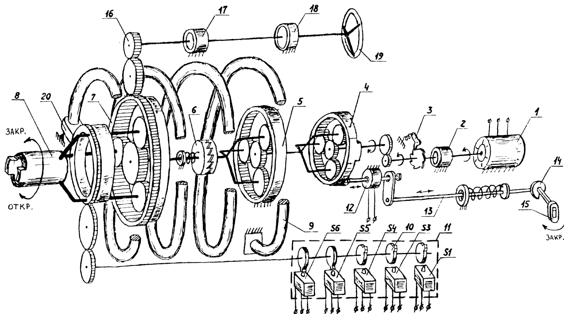
Кинематическая схема механизма МБОВ-63/1-0,25(У)
