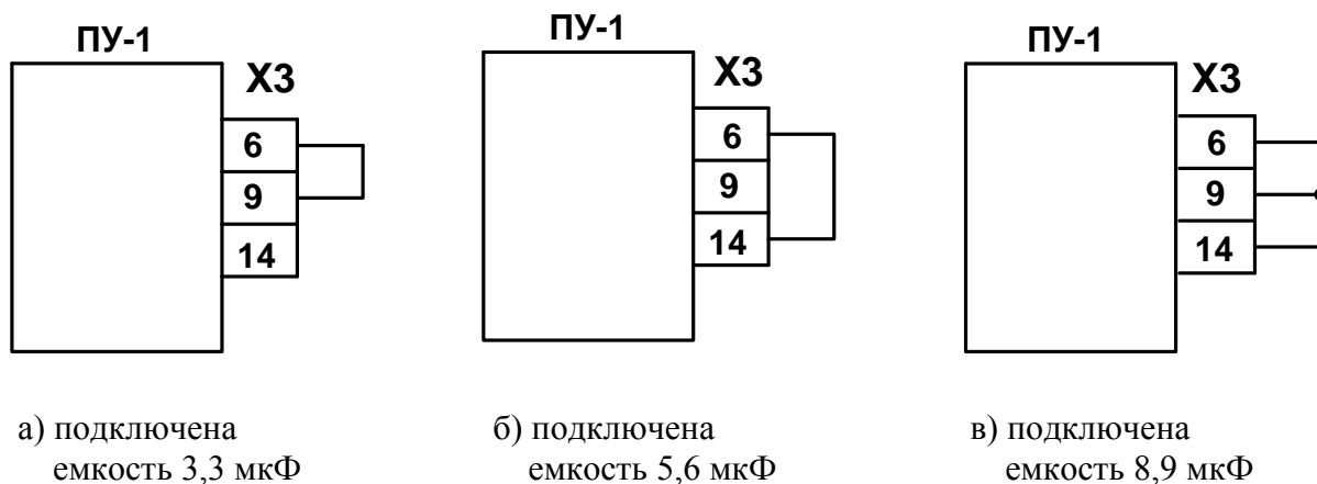
Рис. 4. Варианты установки перемычек для выбора величины ёмкости фазосдвигающего конденсатора
